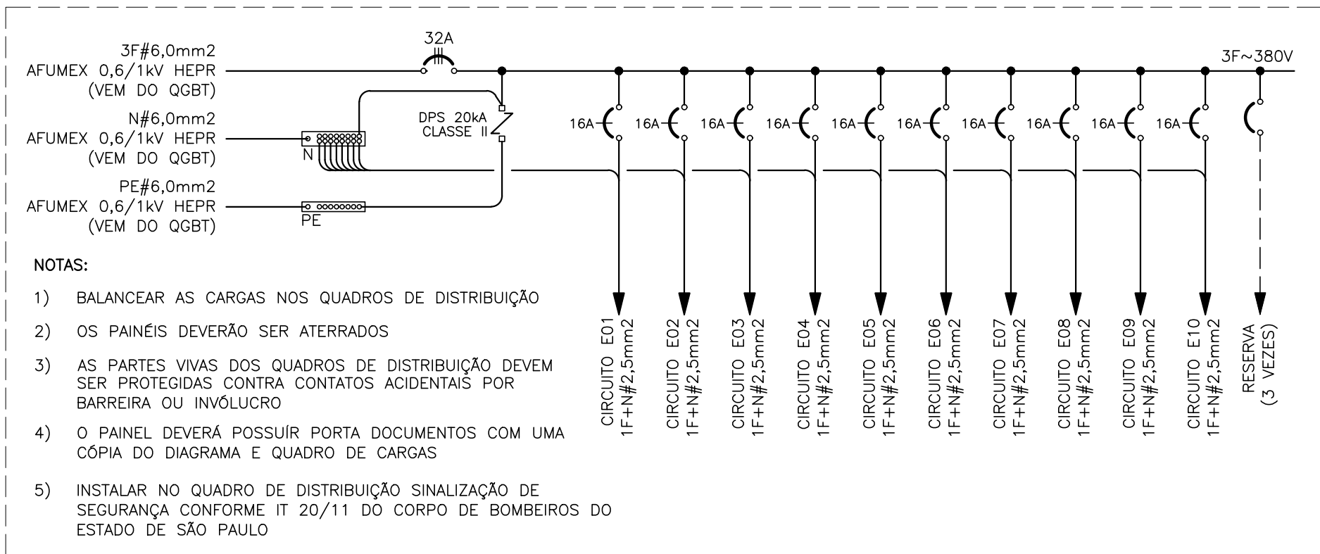
DIAGRAMA UNIFILAR DO QD1
