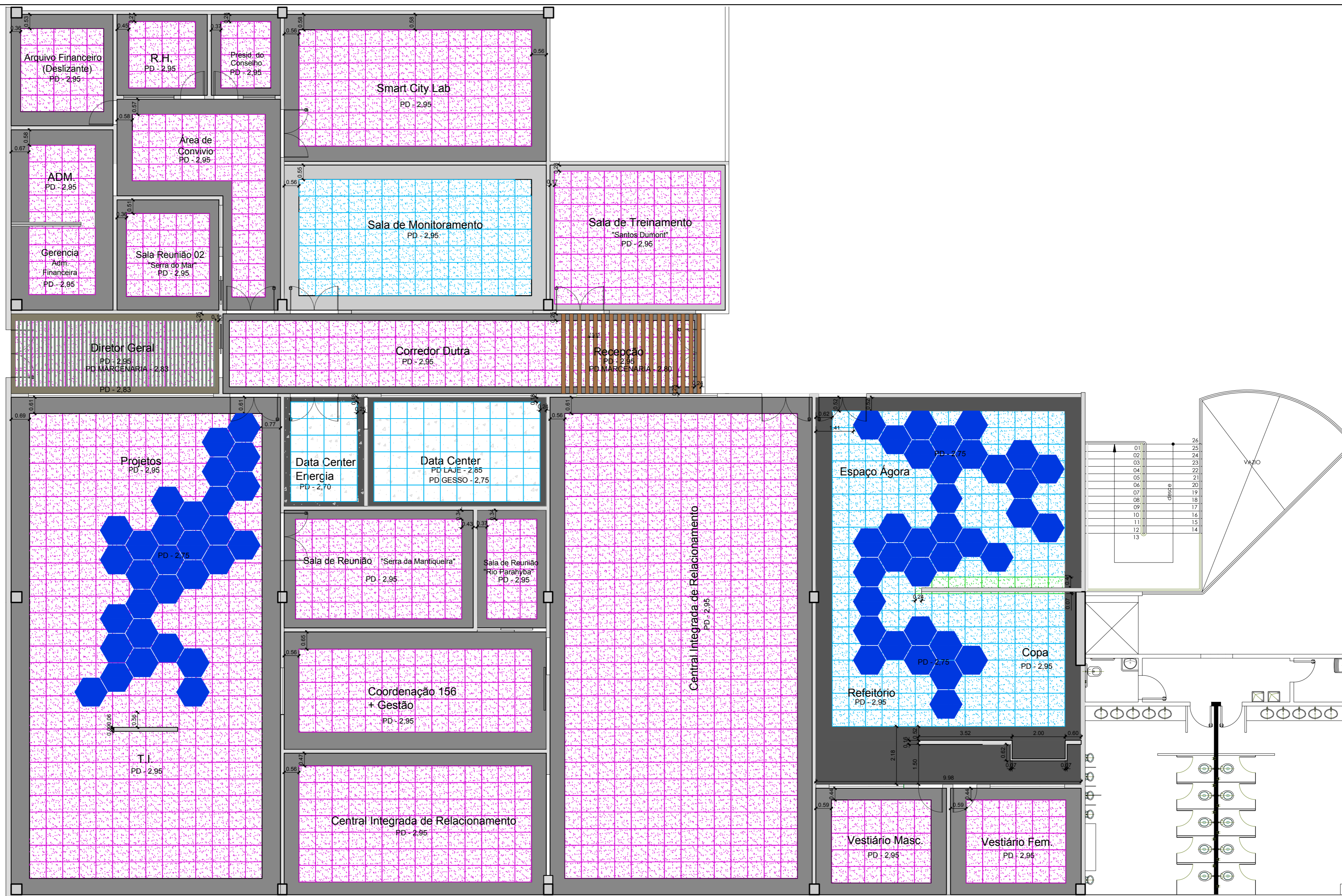
PLANTA DO PAVIMENTO SUPERIOR - PARQUE TECNOLÓGICO DE SÃO JOSÉ DOS CAMPOS - CENTRO EMPRESARIAL II PLANTA DE FORRO ESCADA 1/100
