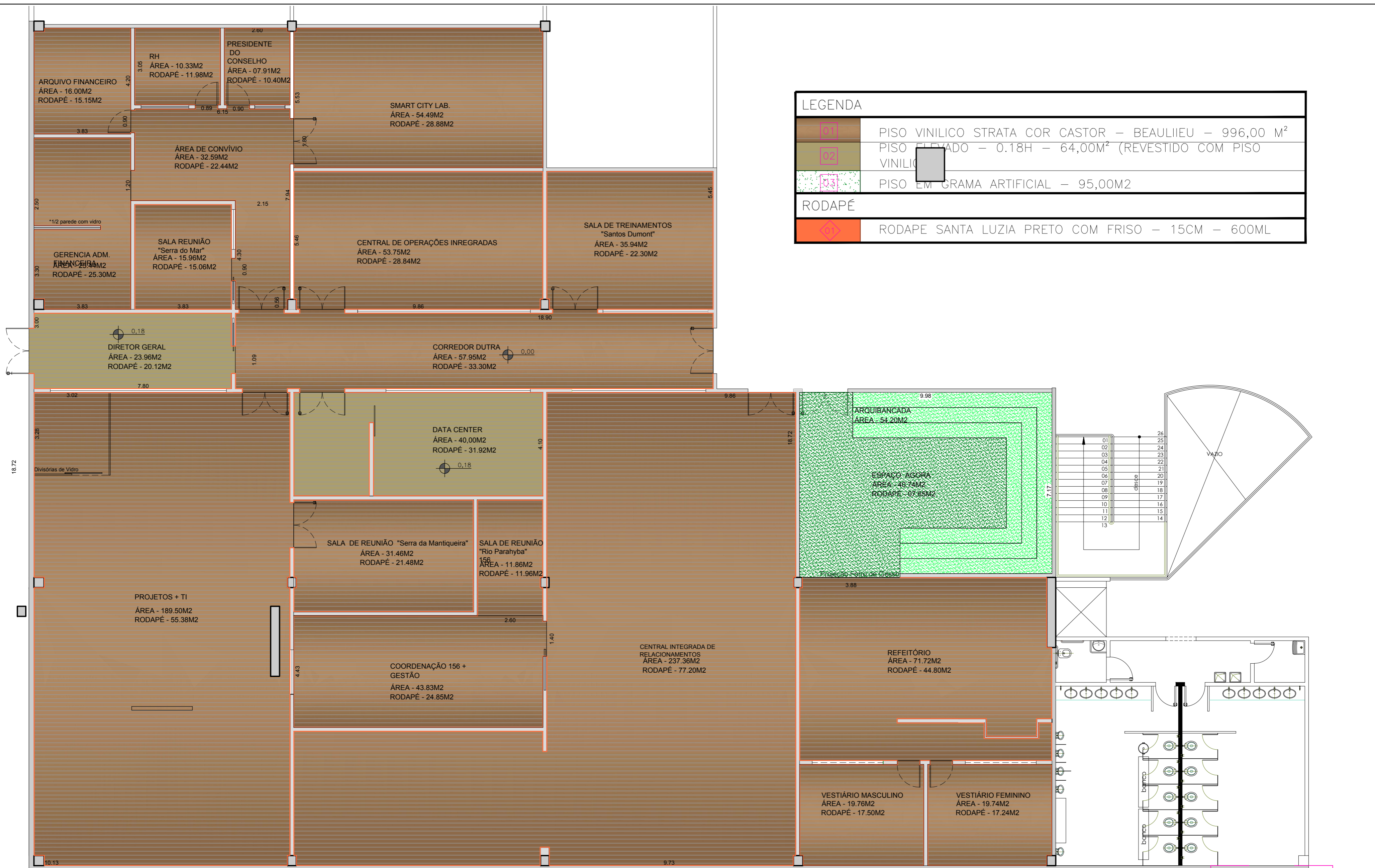
PLANTA DO PAVIMENTO SUPERIOR - PARQUE TECNOLÓGICO DE SÃO JOSÉ DOS CAMPOS - CENTRO EMPRESARIAL II PLANTA DE PISO E RODAPÉ
